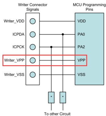
图 1. 烧录引脚连接
