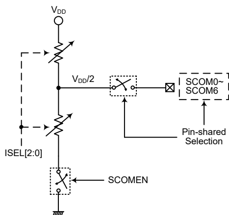
软件控制的 LCD 驱动结构
