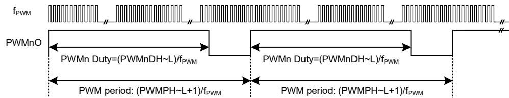
PWM 时序图
