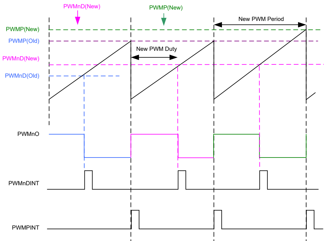
PWM 时序图
