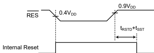
\overline{\text{RES}} 复位时序图
