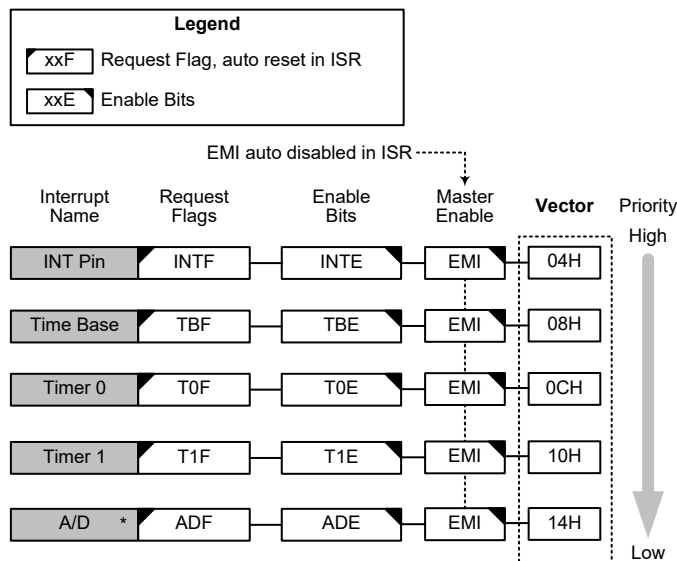
中断结构
