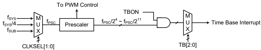
时基中断
