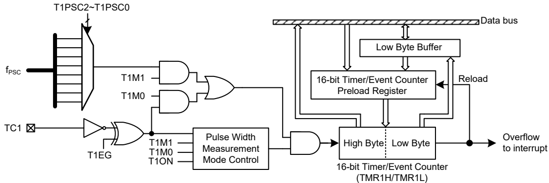
16-bit 定时 / 事件计数器结构
