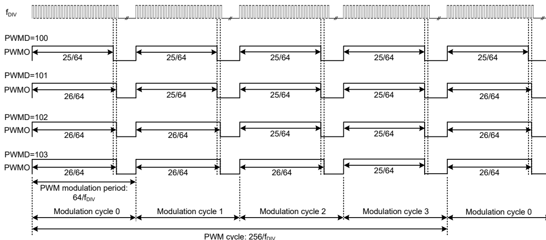
(6+2) 位 PWM 模式调制波形
