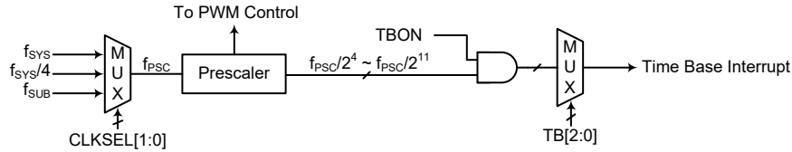
时基中断
