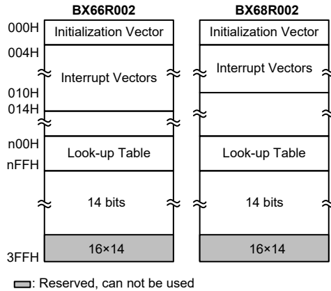
程序存储器结构
