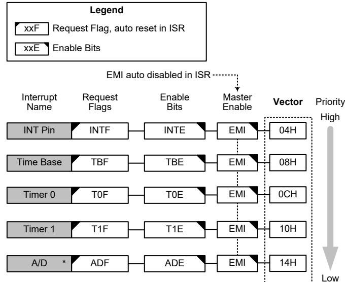
中断结构
