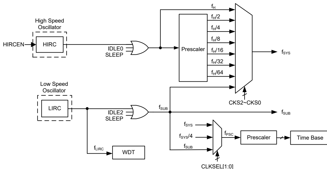
单片机时钟选项
