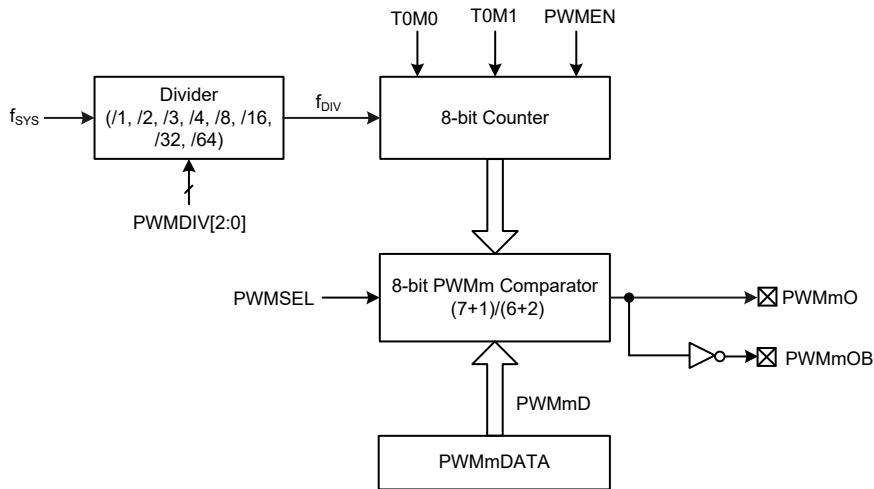
PWM 模式方框图
