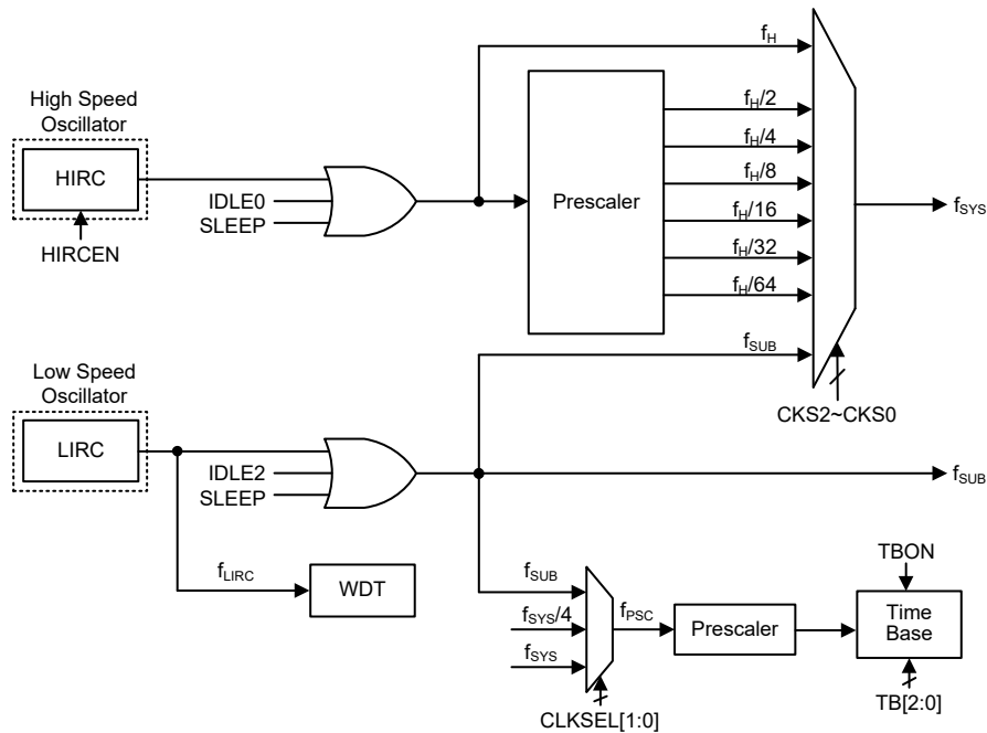
单片机时钟选项
