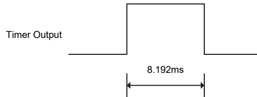
定时器输出 - f_H=4\text{MHz} , T[8:0]=511
